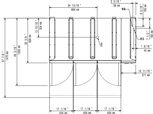
Planta
