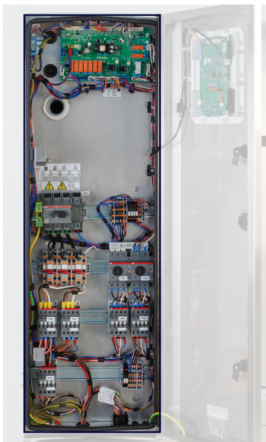
Conexión eléctrica en un solo punto
