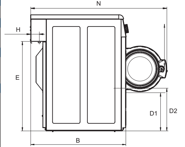
Yandan görünüm
