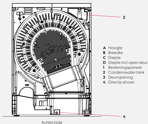
Achterzijde
