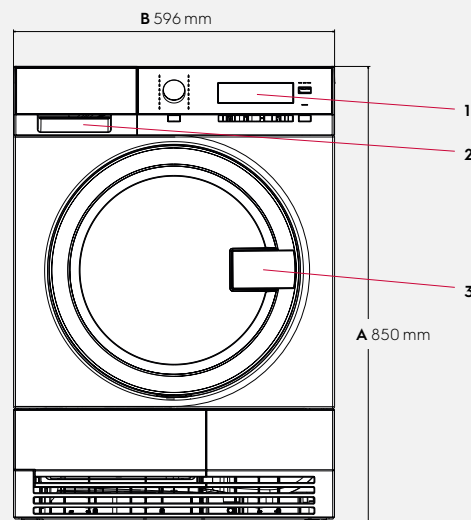
Voorzijde
