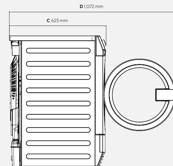
Rechterzijde
