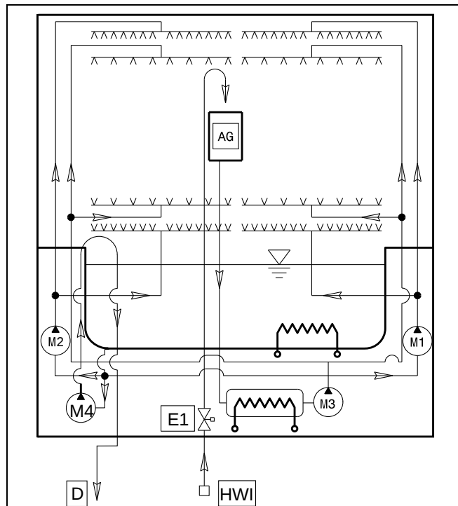
EPPWEL (elektrisk version) utan avloppspump
