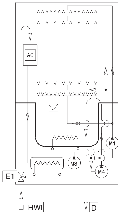
Hydraulkretsritning för EPPWEL (elektriska versioner)
