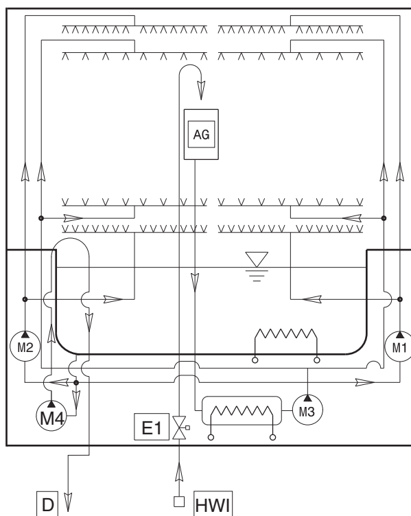
Hydraulkretsritning för EPPWEL (elektriska versioner)
