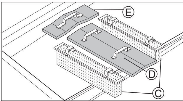
Figur 23 Brunnsfilter
