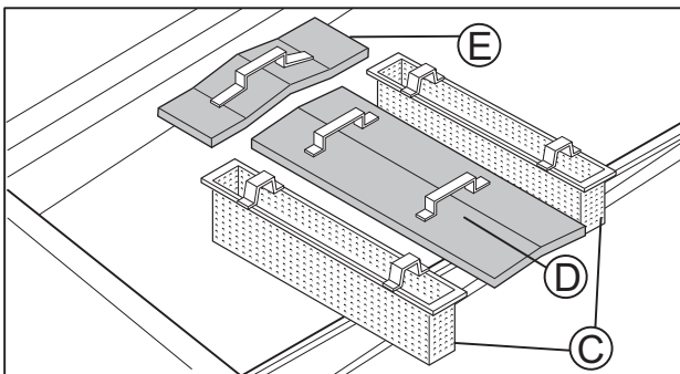
Figure 24 Filtres de cuve
