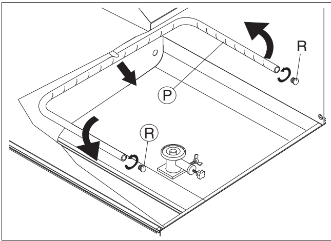
Figure 27 Démontage des bras de lavage fixes
