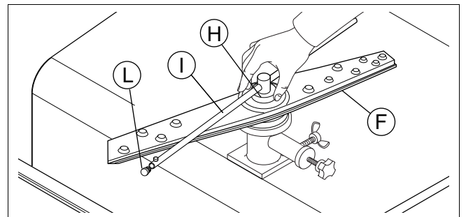
Figure 26 Bras de lavage tournants et bras de rinçage
