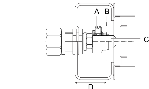
Fig. 1 – Brûleur principal injecteur
