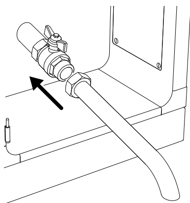
Fig. 1 Rallonge d'arrivée d'huile
