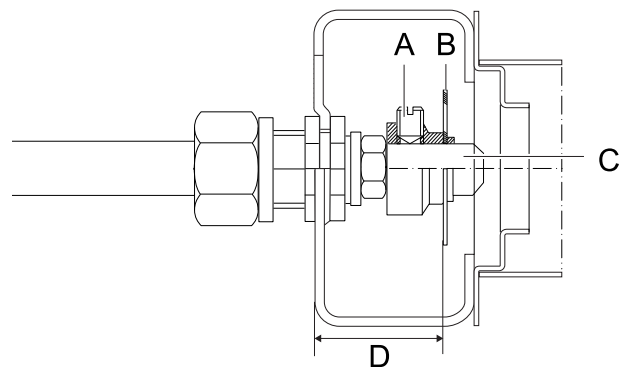
Fig. 1 – Hauptbrennerdüse
