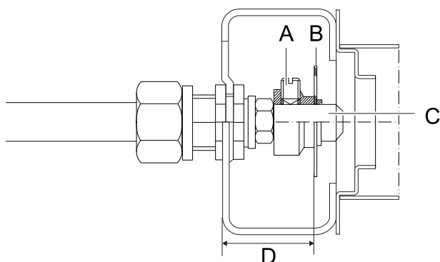
Fig. 1 – Hauptbrennerdüse
