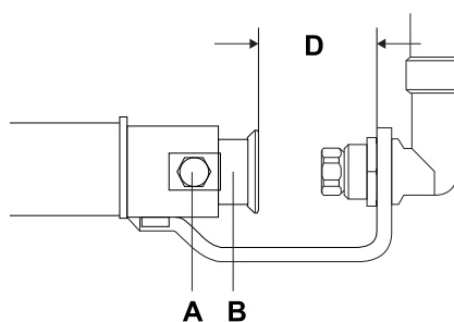
Fig. 1 – Brûleur principal injecteur
