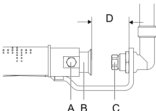
Fig. 1 – 主燃烧器喷嘴
