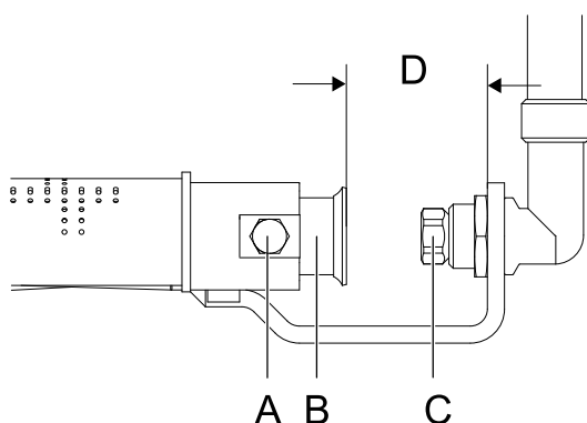
Fig. 1 – Inyector del quemador principal
