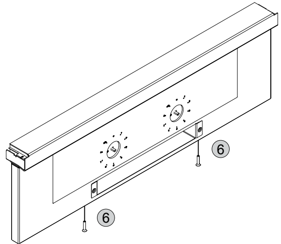
Zugang zur Netzstromversorgung
