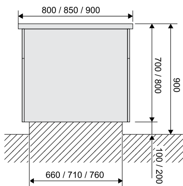
2. Sur un socle en béton
