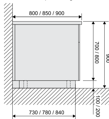
3. Contre un mur, sur un socle en acier ou des pieds réglables
