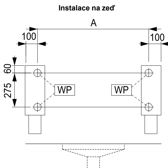
WP = body upevnění na zeď
