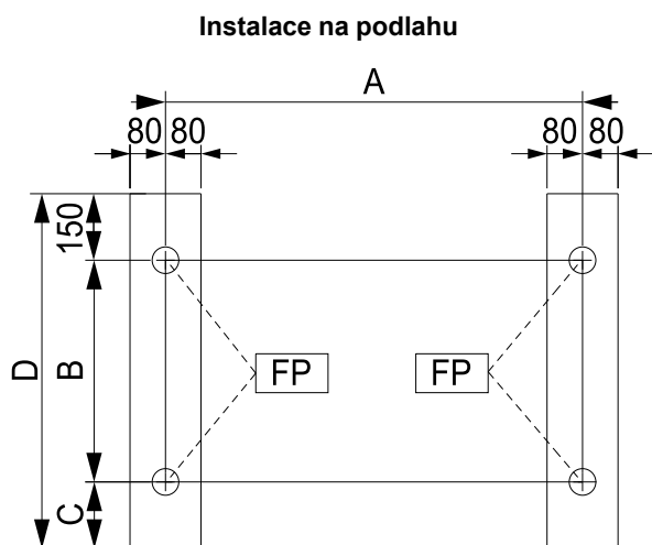
FP = body upevnění na podlahu
