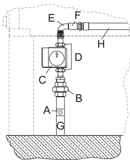
Apparecchiature montate a pavimento
