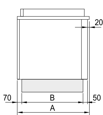
Montage autonome
