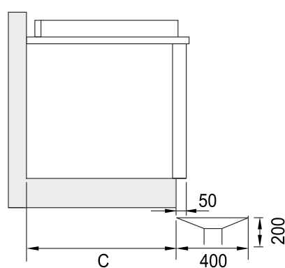
Montage mural
