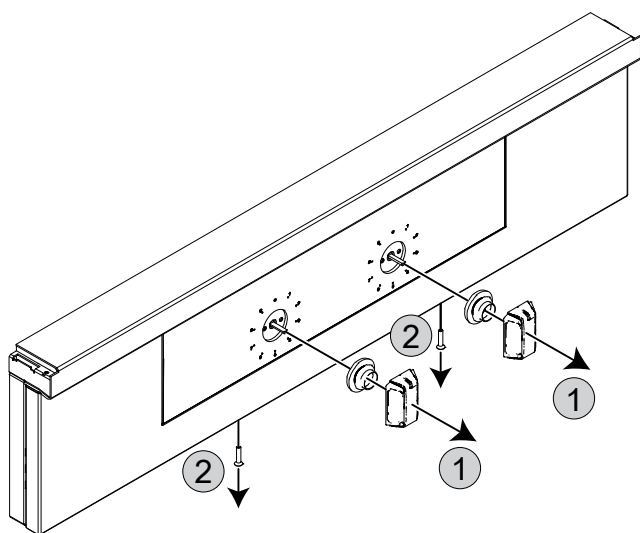
Tillträde till strömförsörjning
