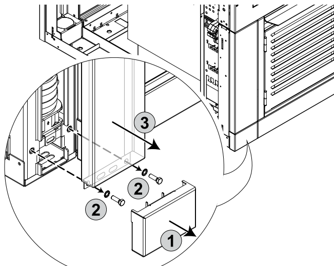
Tillträde till strömförsörjning för marinversion, bredd 500 mm
