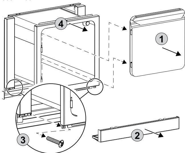
Tillträde till strömförsörjning för marinversion, bredd 800/1 200 mm
