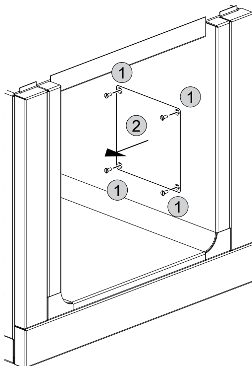
Tillträde till strömförsörjning för marinversion, bredd 800/1 200 mm
