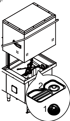
Abbildung 25 Filter
