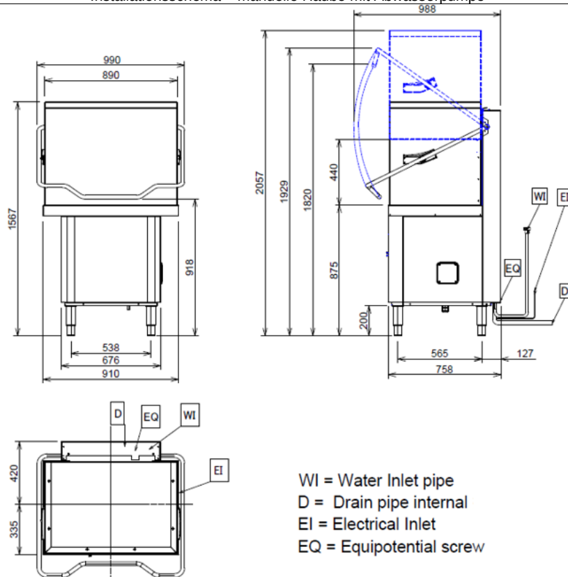
Installationsschema – manuelle Haube mit Abwasserpumpe
