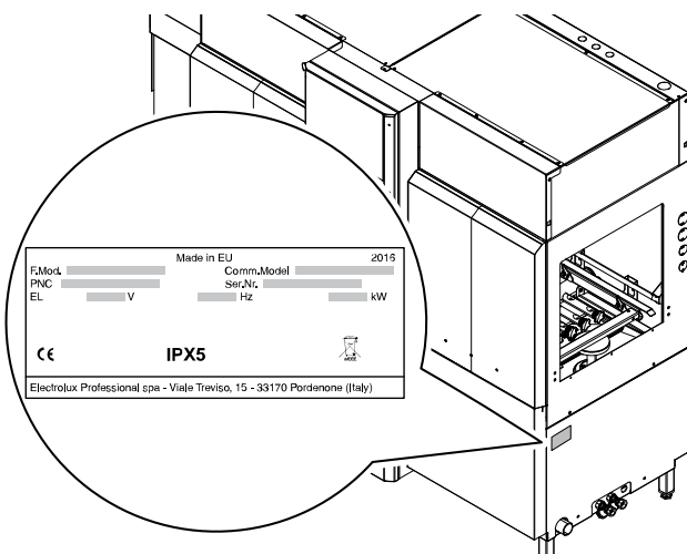
Fig. 2 Märklattans placering (maskinens vänstra sida)
