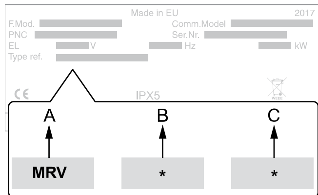
Fig. 2 Märklattans placering (maskinens vänstra sida)
