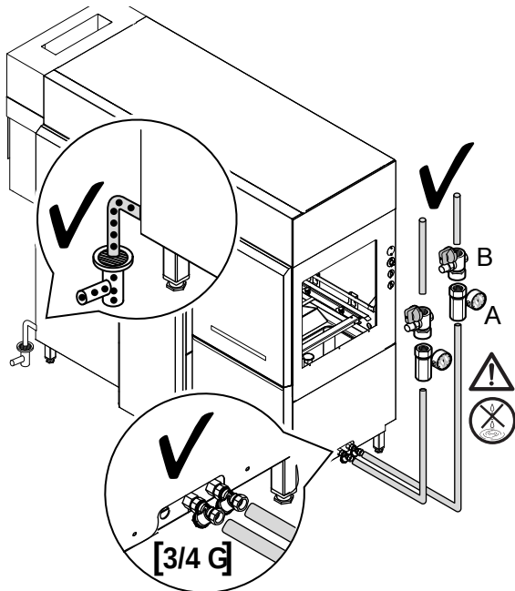
Fig. 4 Aansluiting waterleiding voor rechtermachine
