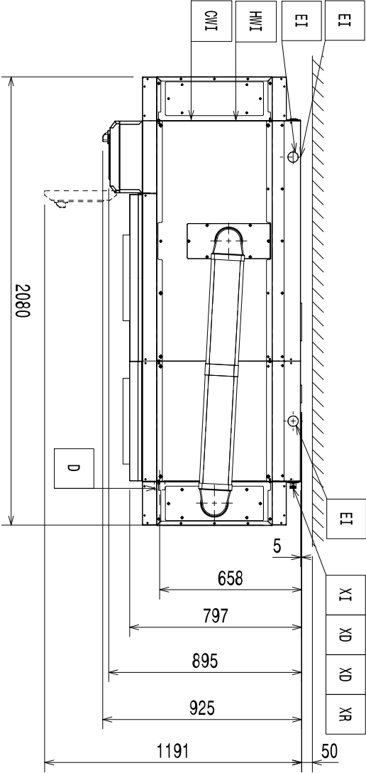
Schéma instalace
