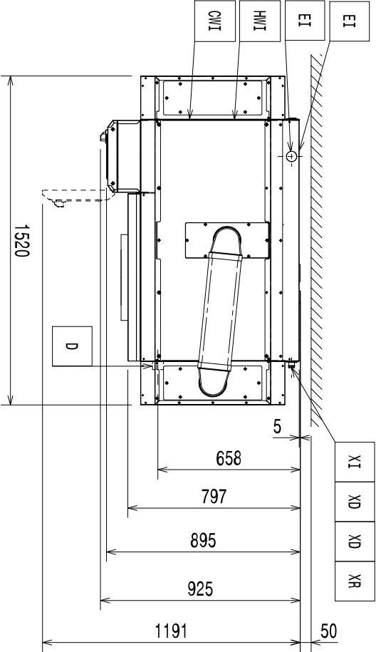
Schéma instalace
