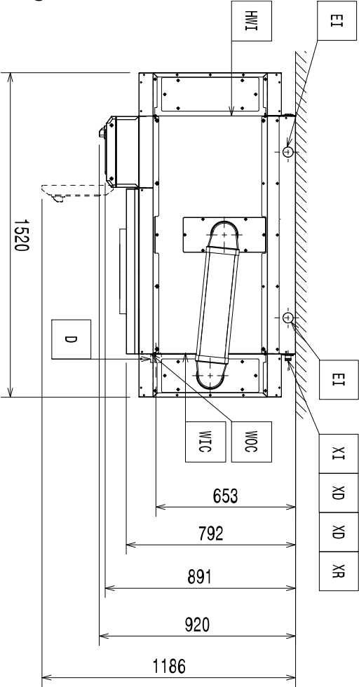
Diagrama de instalación
