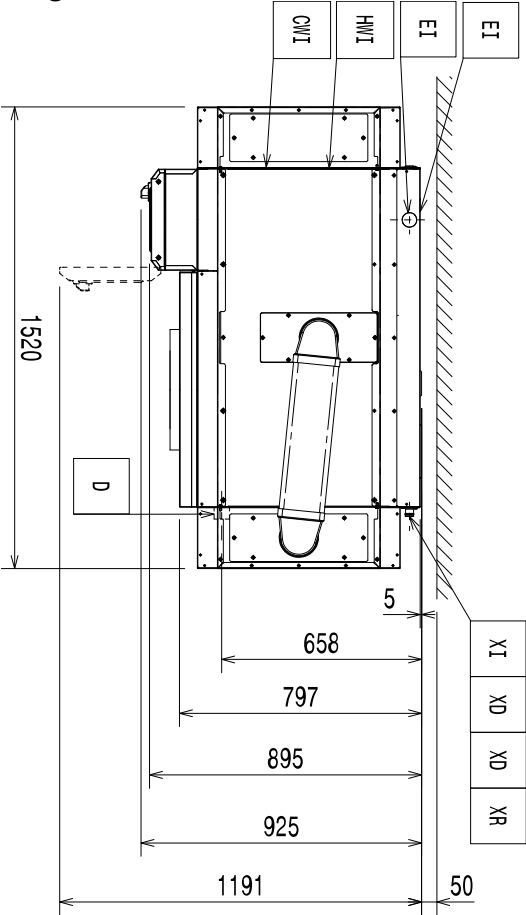
Diagrama de instalación
