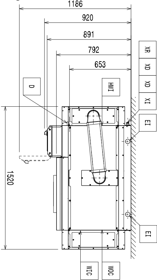
Diagrama de instalación
