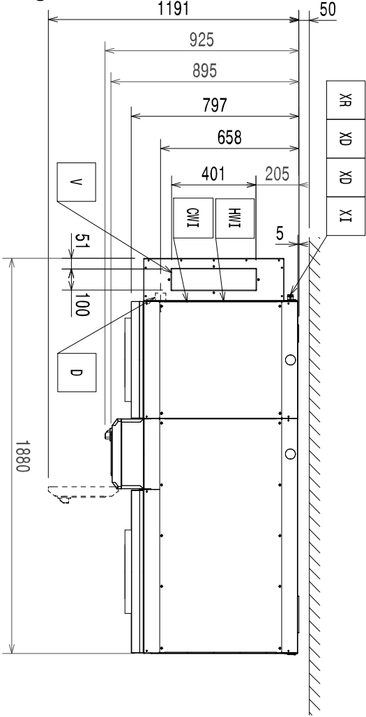
Diagrama de instalación
