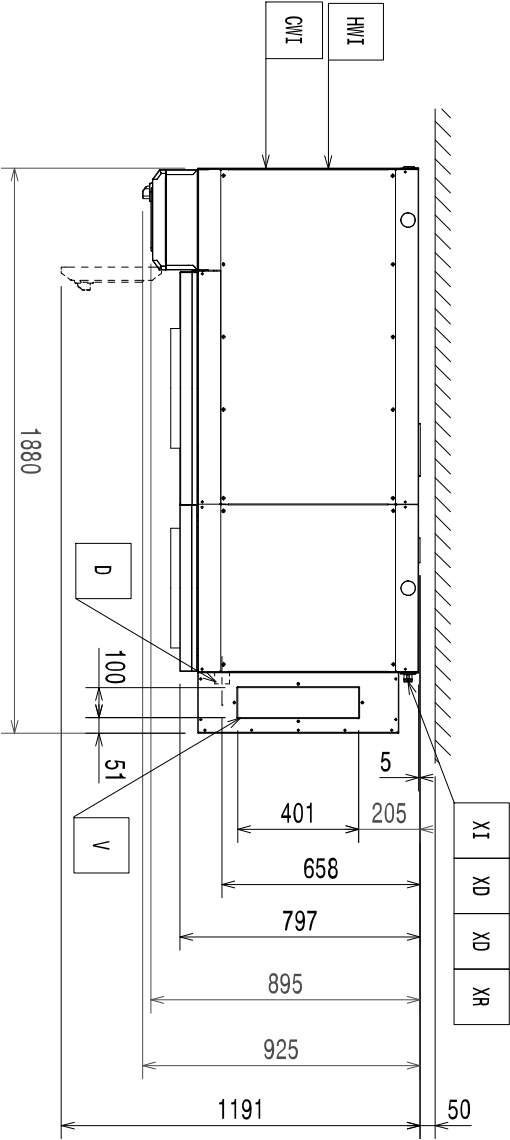
Diagrama de instalación
