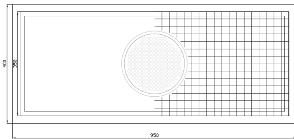
Boven aanzicht
