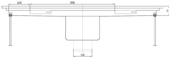
Front aanzicht
