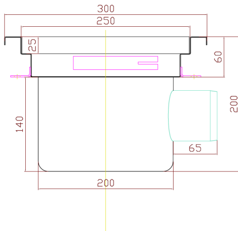
Front aanzicht
