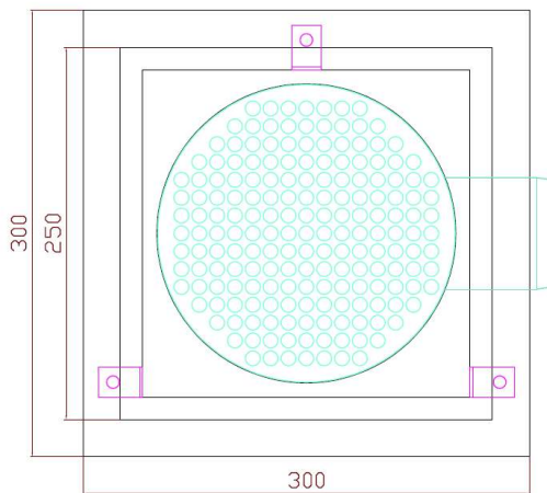
Boven aanzicht
