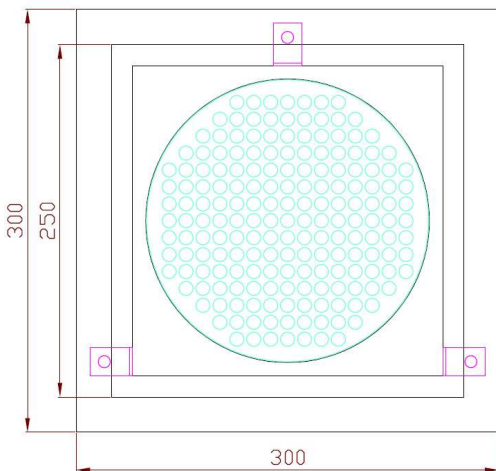
Boven aanzicht
