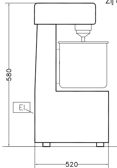
Zij aanzicht
