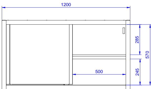
Front aanzicht
