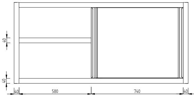
Zij aanzicht
