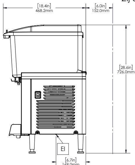
Zij aanzicht
