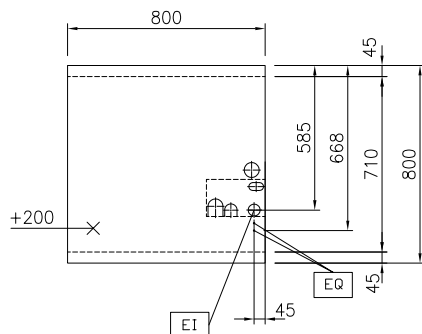
Boven aanzicht
