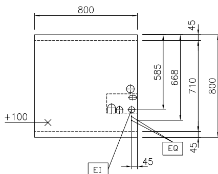
Boven aanzicht
