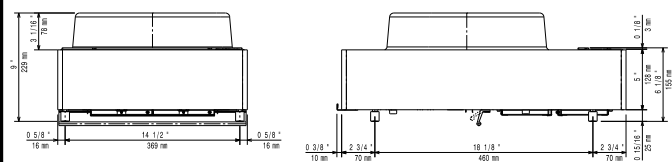
Oldalnézet
