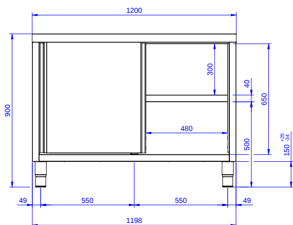
Fronte
