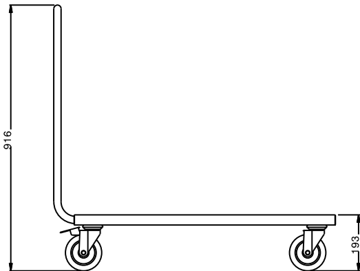
Avant
