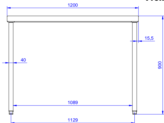
Fronte
