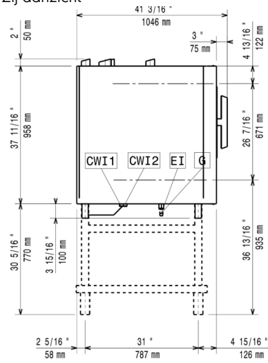
Zij aanzicht
