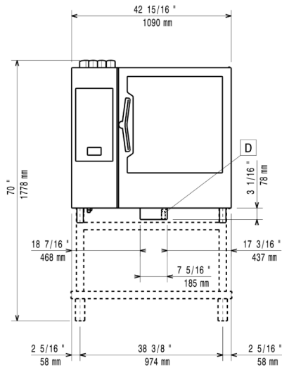
Front aanzicht
