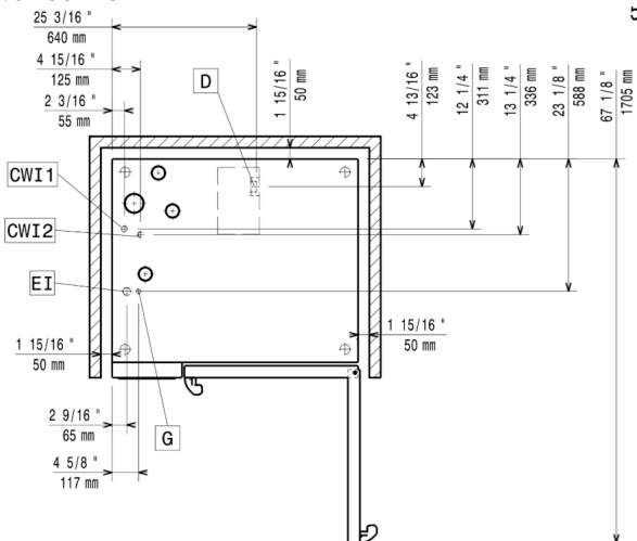
Boven aanzicht
