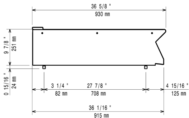
Zij aanzicht
