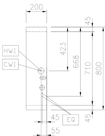
Boven aanzicht
