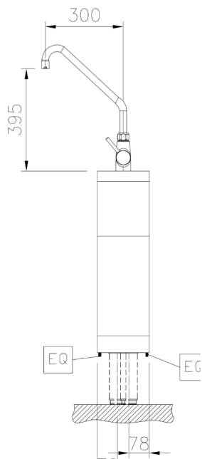
Front aanzicht
