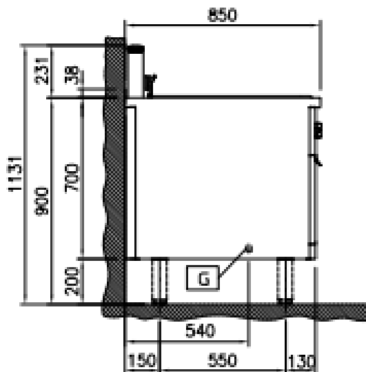
Zij aanzicht
