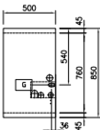
Boven aanzicht
