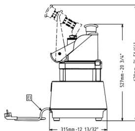
Zij aanzicht
