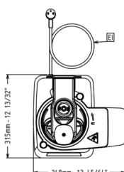
Boven aanzicht
