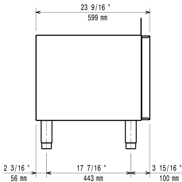
Côté
