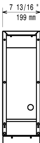
Dessus
