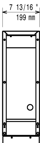
Dessus
