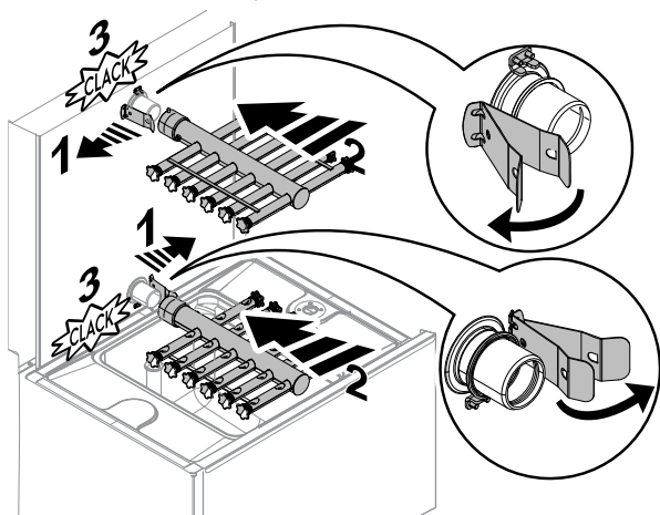
2. brazos de prelavado y lavado del módulo de 35";
