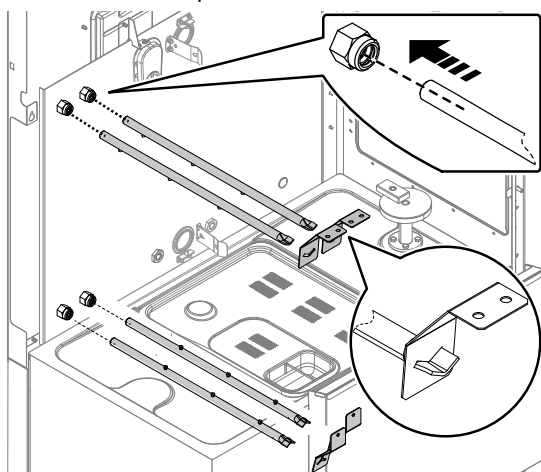
3. bracci del modulo risciacquo.
