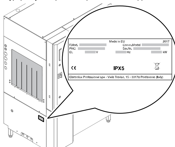
Fig. 1 Plaats van het typeplaatje
