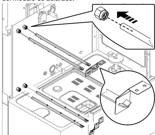
3. brazos del módulo de aclarado.
