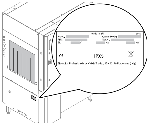
Kuva 1 Tyyppikilven sijainti
