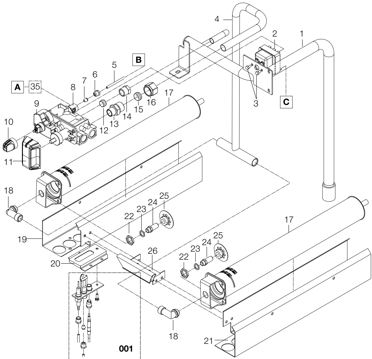
001 - DETAIL ZÜNDBRENNER
