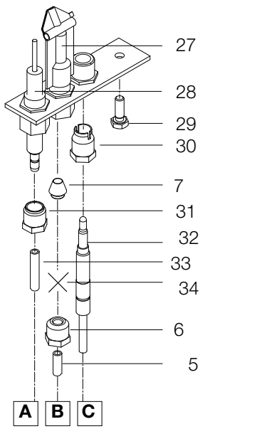
001 - DETAIL ZÜNDBRENNER
